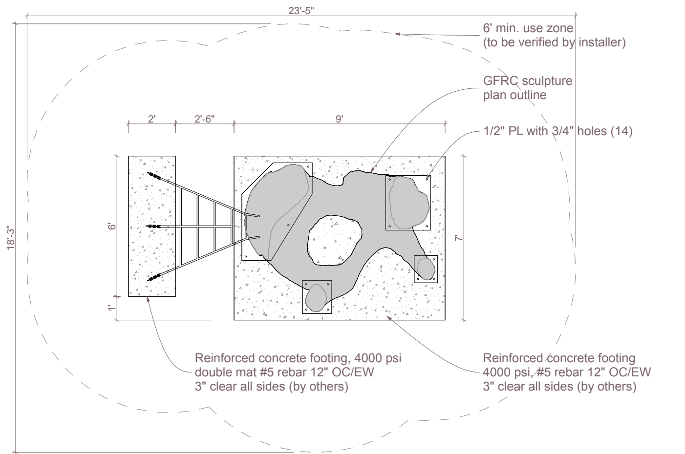
1 Plan SCALE: 1/4" = 1'-0"
