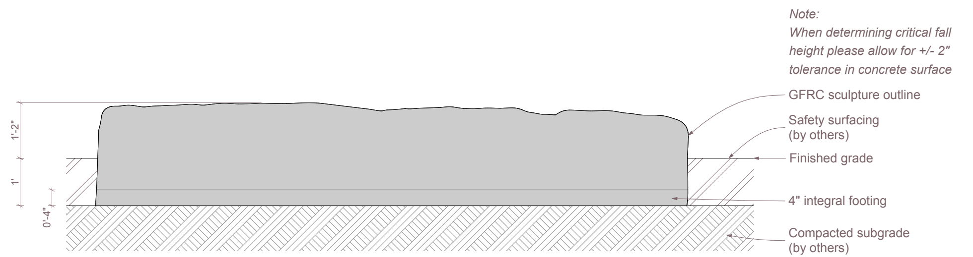
3 Section SCALE: 1/2" = 1'-0"
