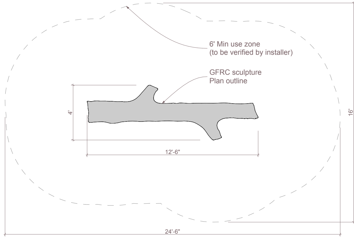
1 Plan SCALE: 1/4" = 1'-0"
