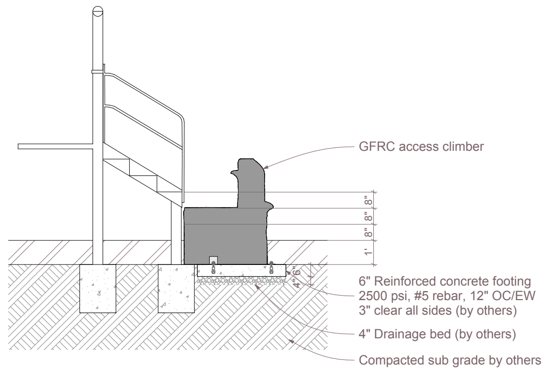
2 Section SCALE: 1/4" = 1'-0"
