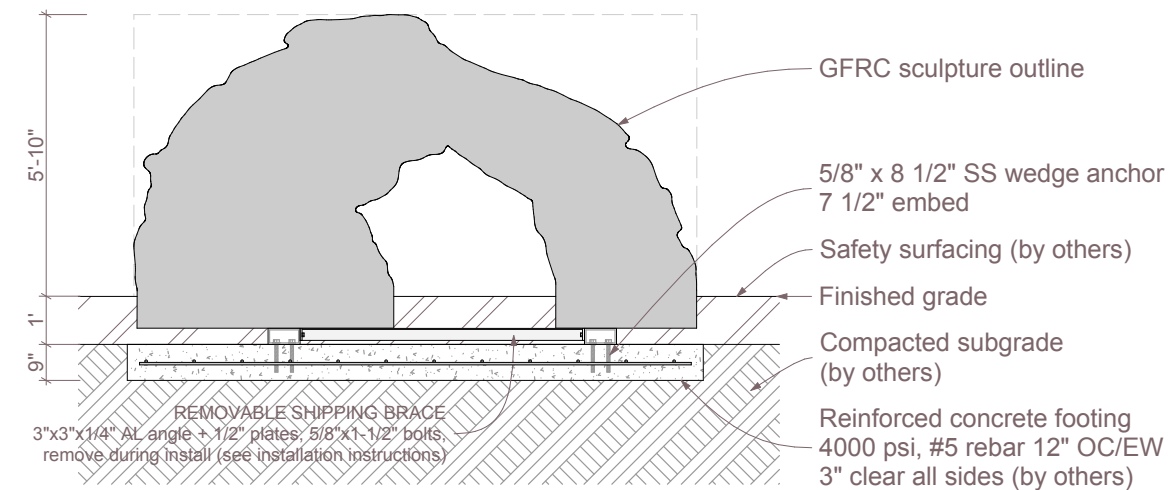
Section SCALE: 1/4" = 1'-0"
