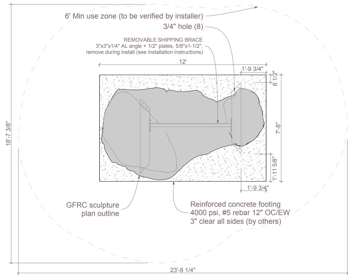
Plan SCALE: 1/4" = 1'-0"
