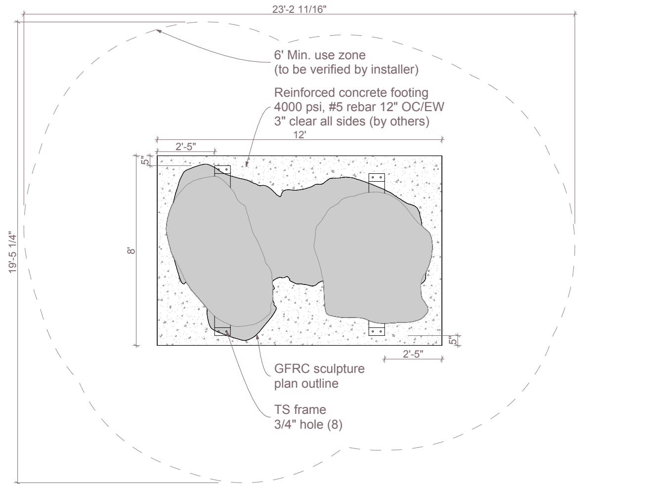
1 Plan SCALE: 1/4" = 1'-0"
