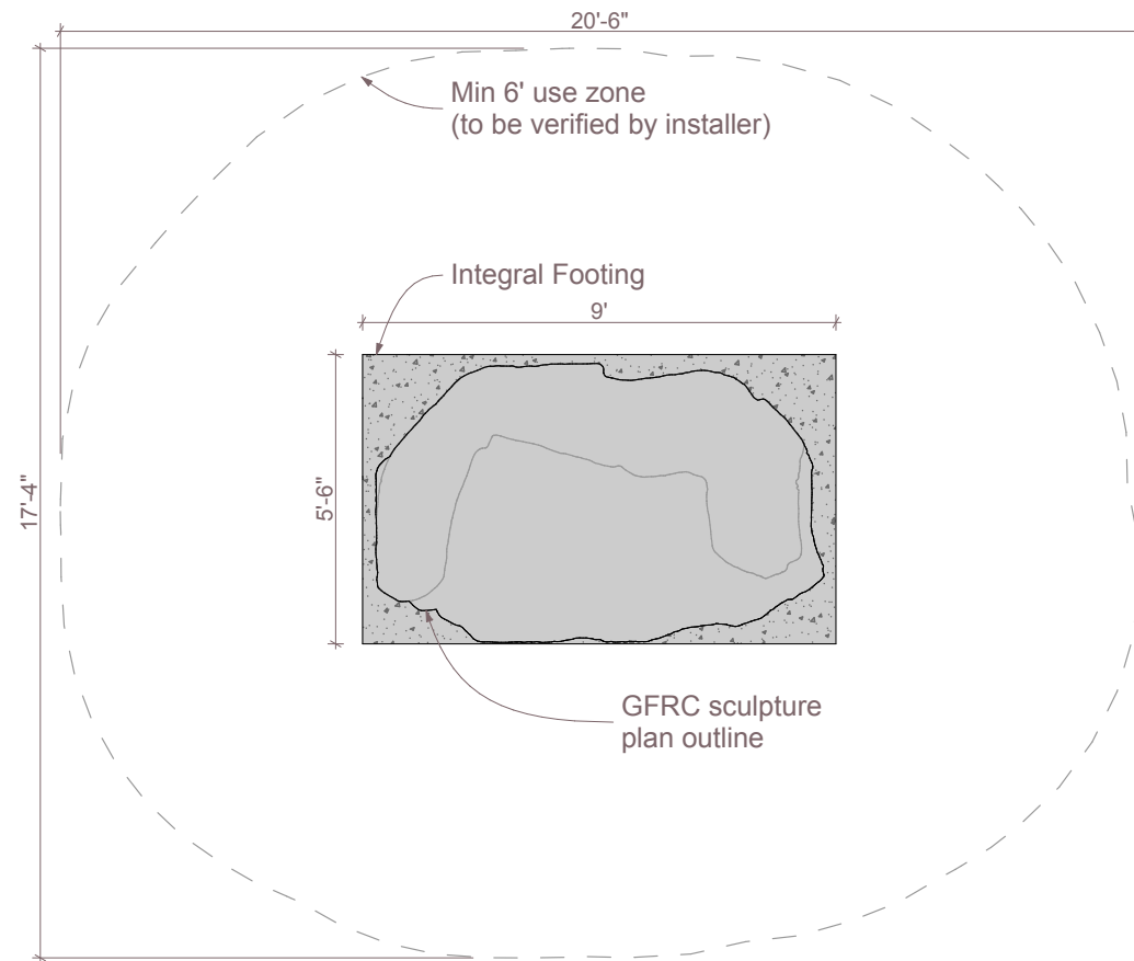
1 Plan SCALE: 1/4" = 1'-0"
