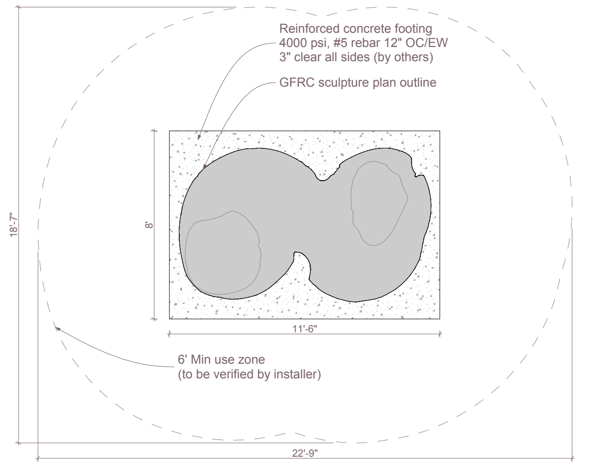
1 Plan SCALE: 1/4" = 1'-0"
