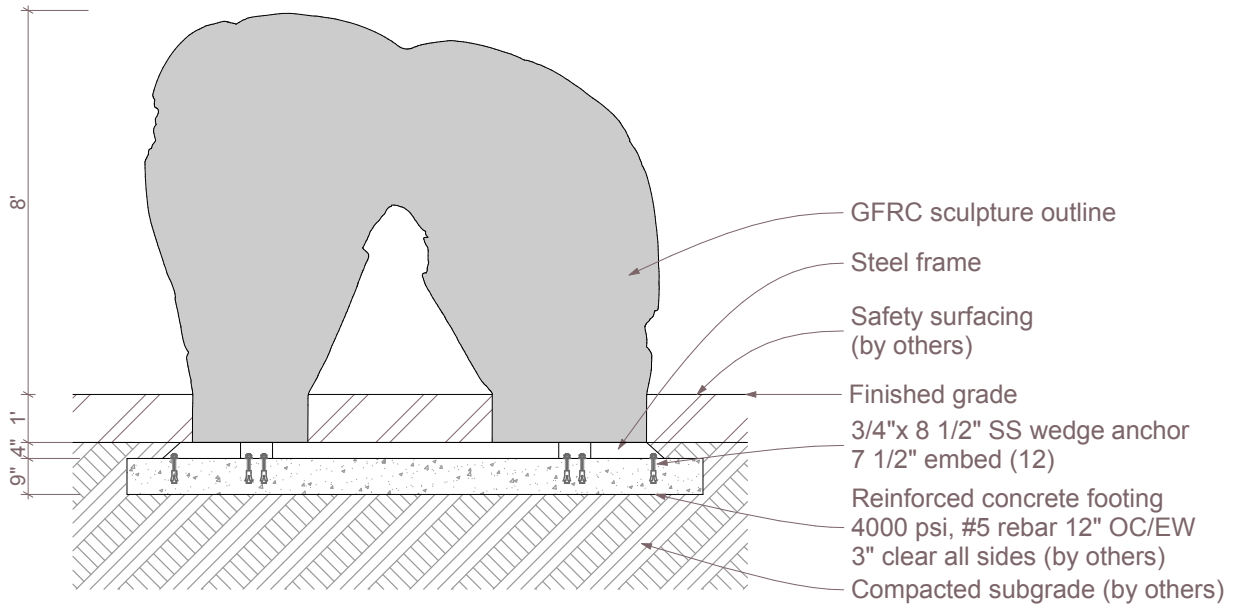
2 Section SCALE: 1/4" = 1'-0"
