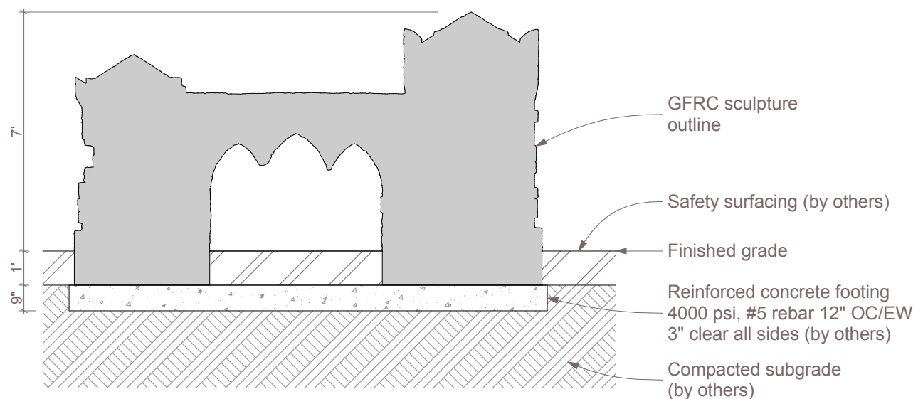
Section SCALE: 1/4" = 1'-0"
