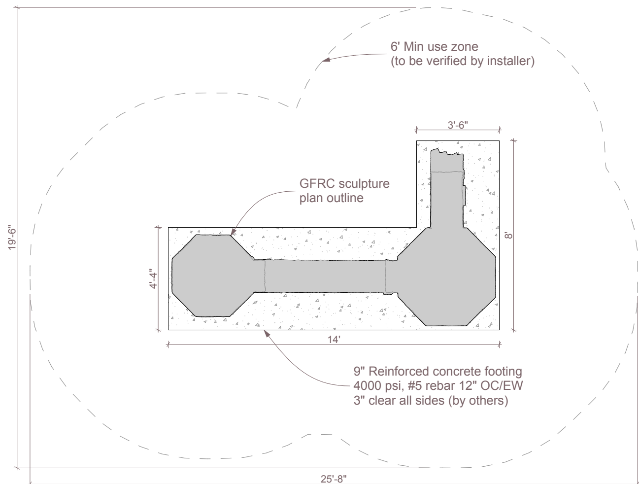
Plan SCALE: 1/4" = 1'-0"
