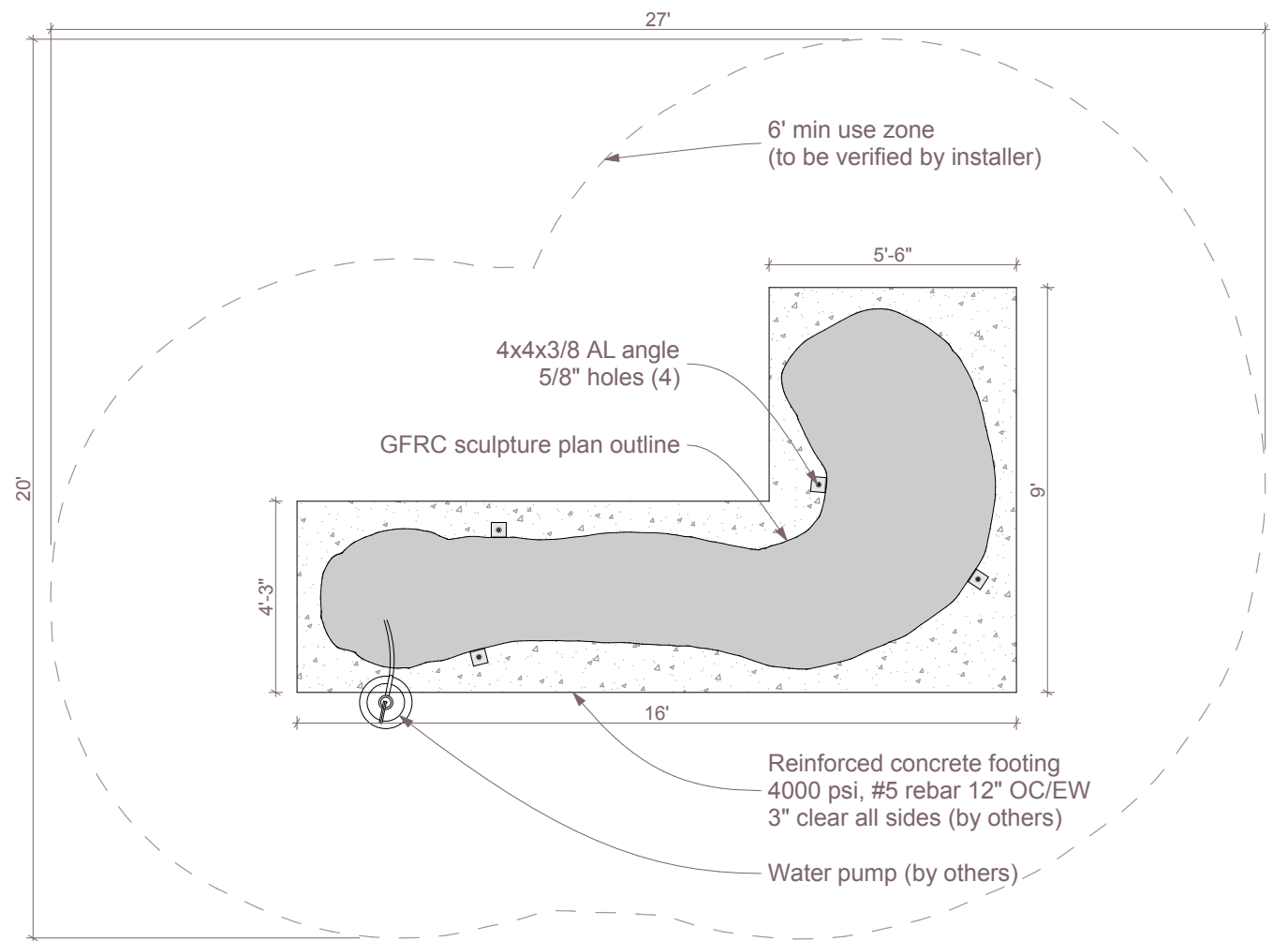
1 Plan SCALE: 1/4" = 1'-0"
