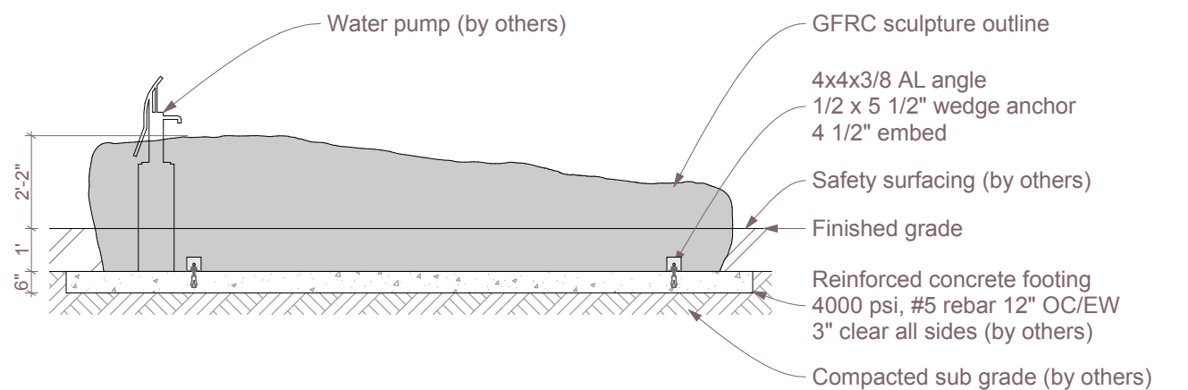
2 Section SCALE: 1/4" = 1'-0"
