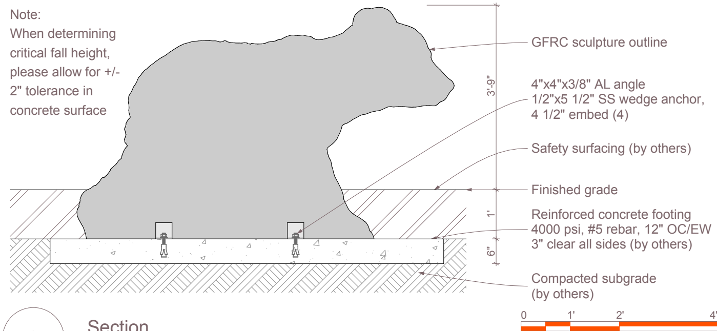
2 Section SCALE: 1/2" = 1'-0"
