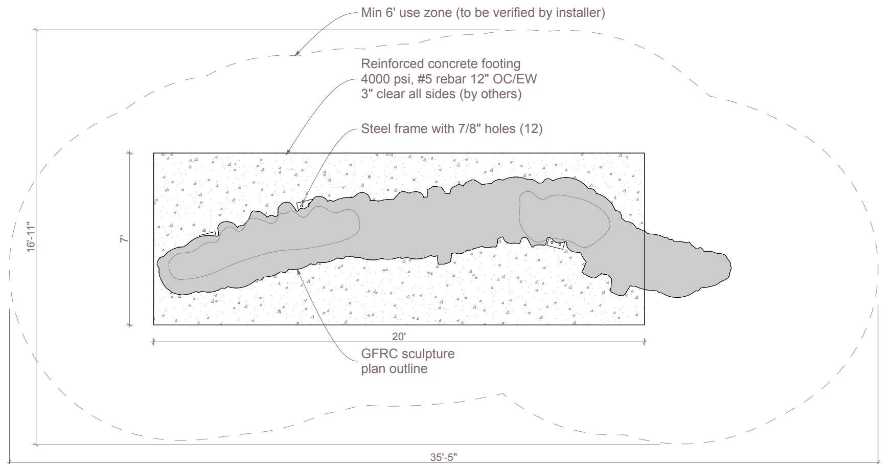
2 Plan SCALE: 1/4" = 1'-0"
