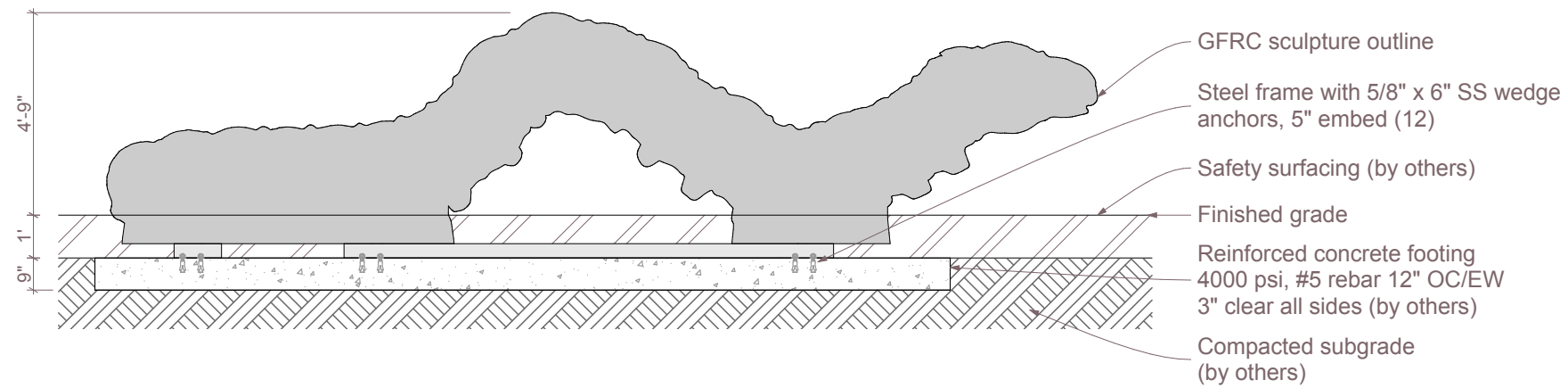
1 Section SCALE: 1/4" = 1'-0"
