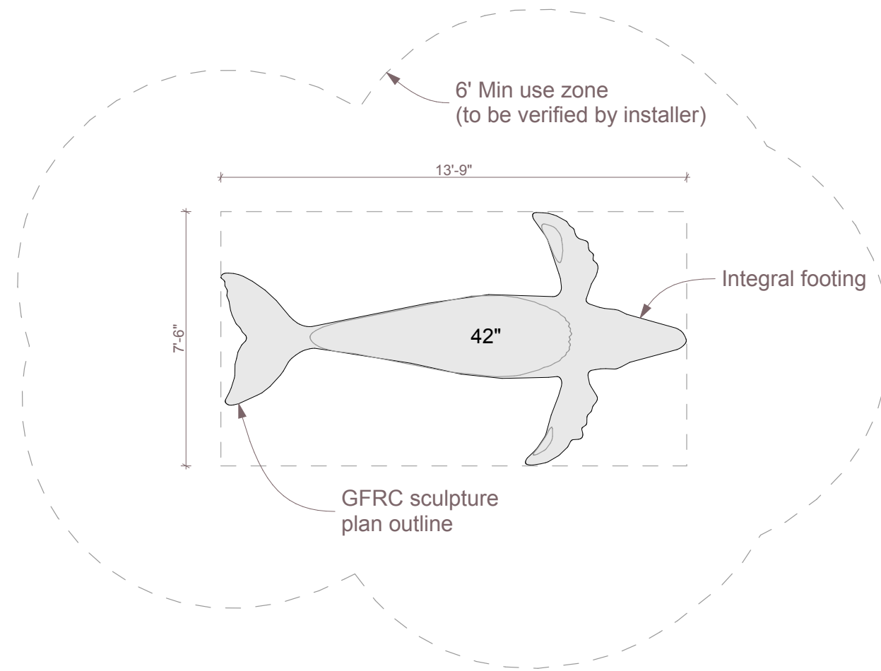
Plan SCALE: 1/4" = 1'-0"
