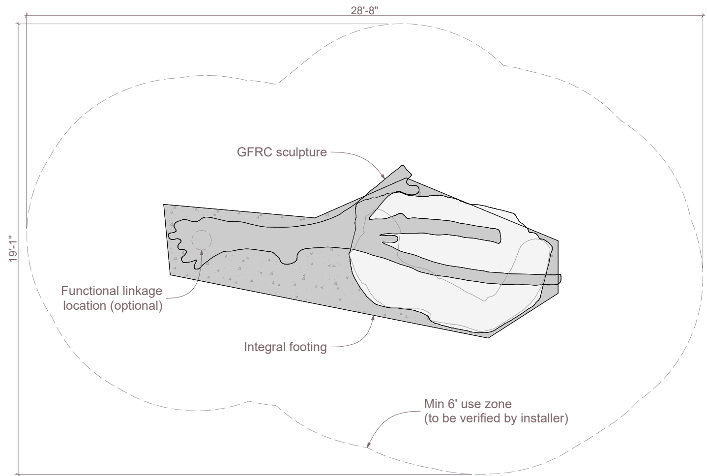
2 Plan SCALE: 1/4" = 1'-0"
