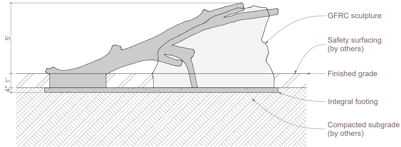
1 Section SCALE: 1/4" = 1'-0"
