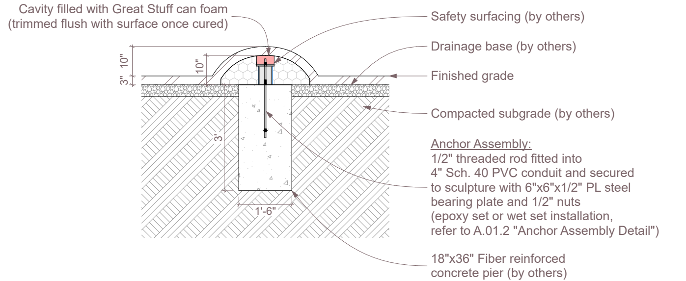
Section SCALE: 3/8" = 1'-0"
