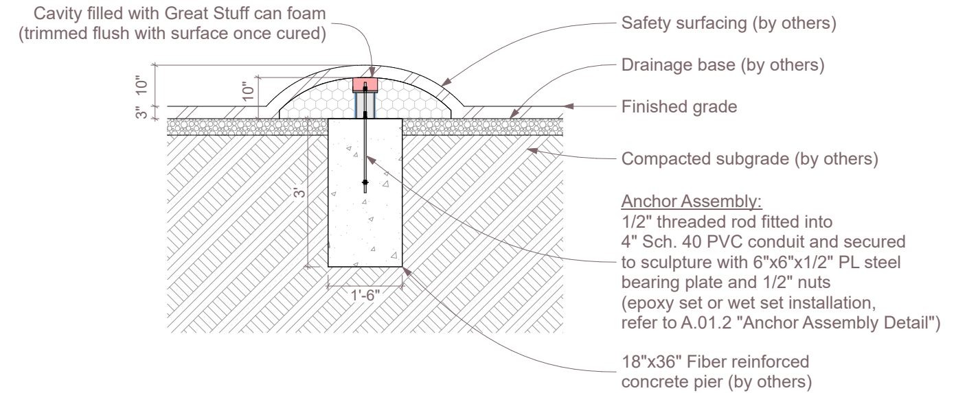
1 Section SCALE: 3/8" = 1'-0"
