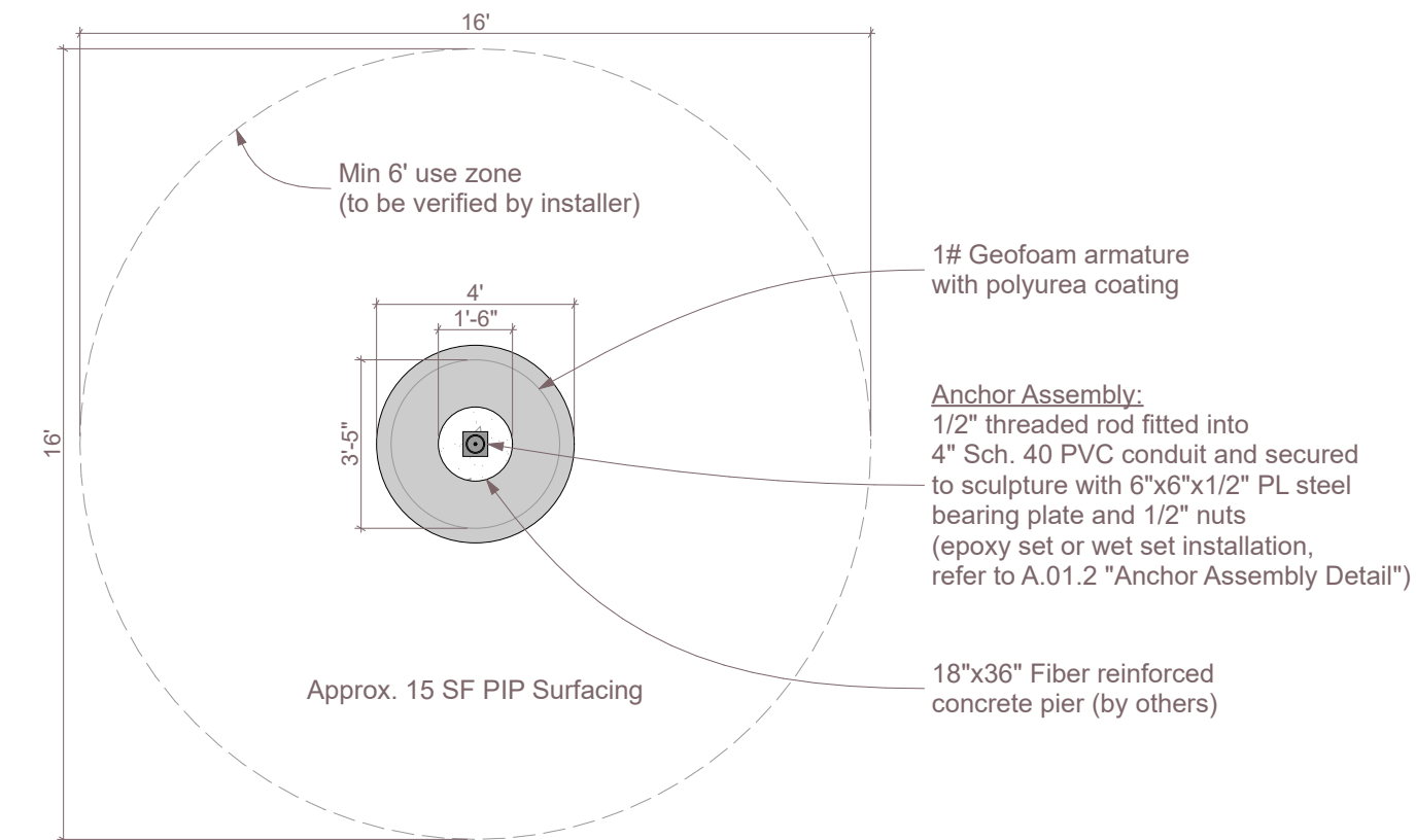
2 Plan SCALE: 1/4" = 1'-0"
